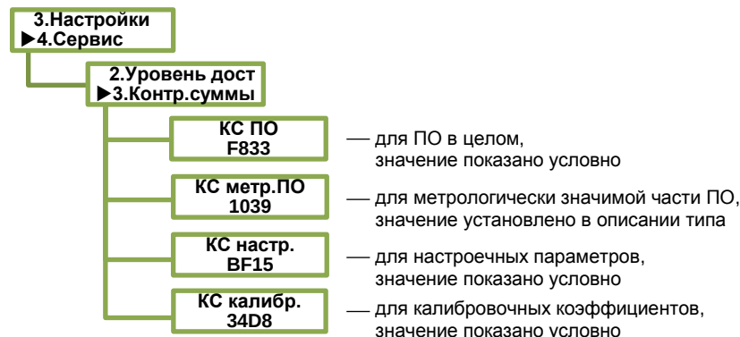
Рисунок 5.14 – Контрольные суммы
