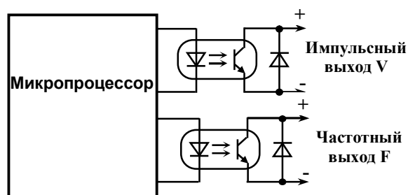
Рисунок 3.3 - Организация выходов преобразователей модификации МФ-Ч
