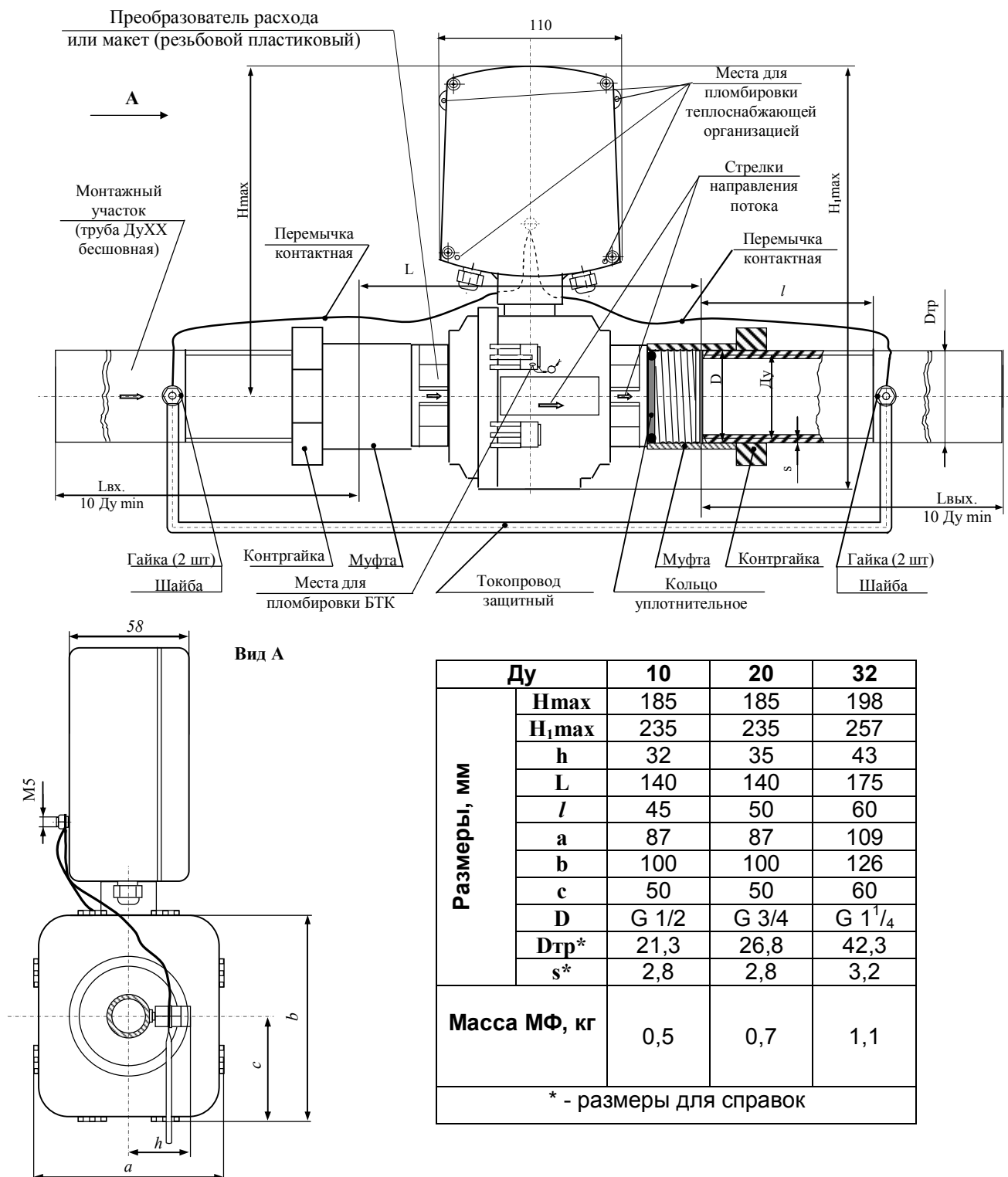
Рисунок А.4 – габаритные и присоединительные размеры преобразователей Ду 10,20,32 исполнений МФ-10.2.1-Э и рекомендации по монтажу
