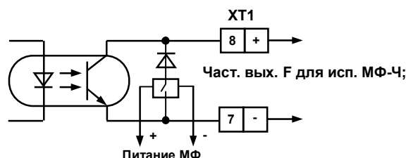
Рисунок В.2 Схема частотного выхода
