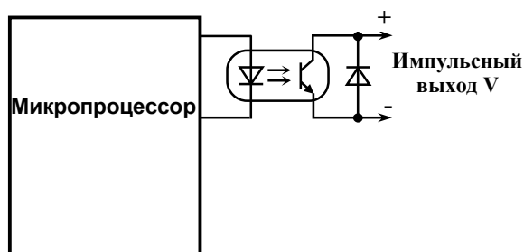
Рисунок 3.2 - Организация выхода преобразователей модификации МФ
