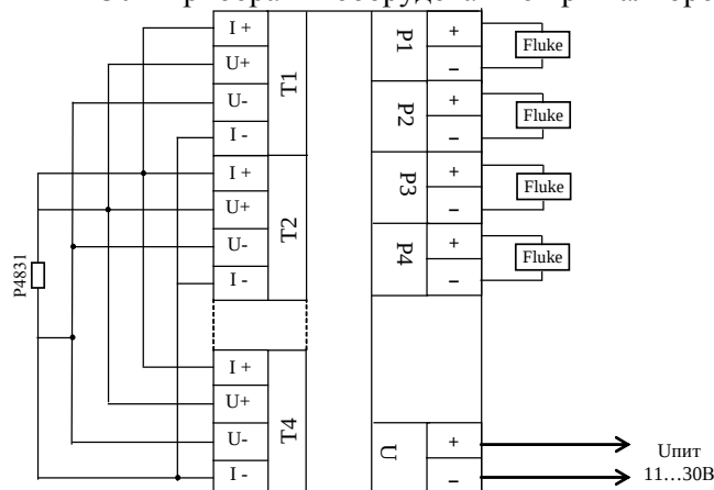
Схема подключения ТМК-Н30 к приборам и оборудованию при калибровке
