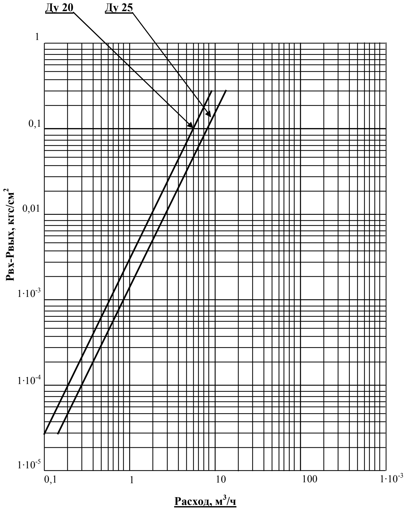
ГРАФИК ПОТЕРЬ НАПОРА (РВХ-РВЫХ) НА ПРЕОБРАЗОВАТЕЛЯХ В ЗАВИСИМОСТИ ОТ РАСХОДА
