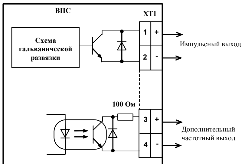
Рисунок Б.1 – Схемы выходных цепей преобразователей ВПС1(2)-ЧИХ.XX
