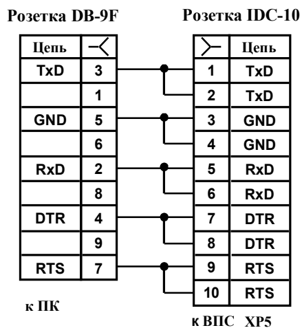
Рисунок Б.2 – Схема кабеля для подключения преобразователей ВПС1(2)-ЧИХ.XX к ПК
