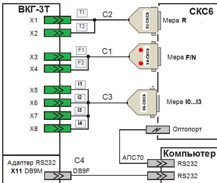
Рисунок 7.1 – Схема поверки
